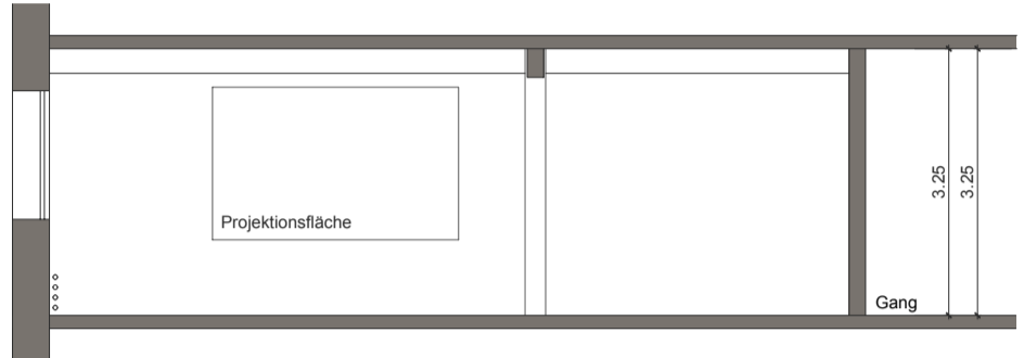
Ansicht B
