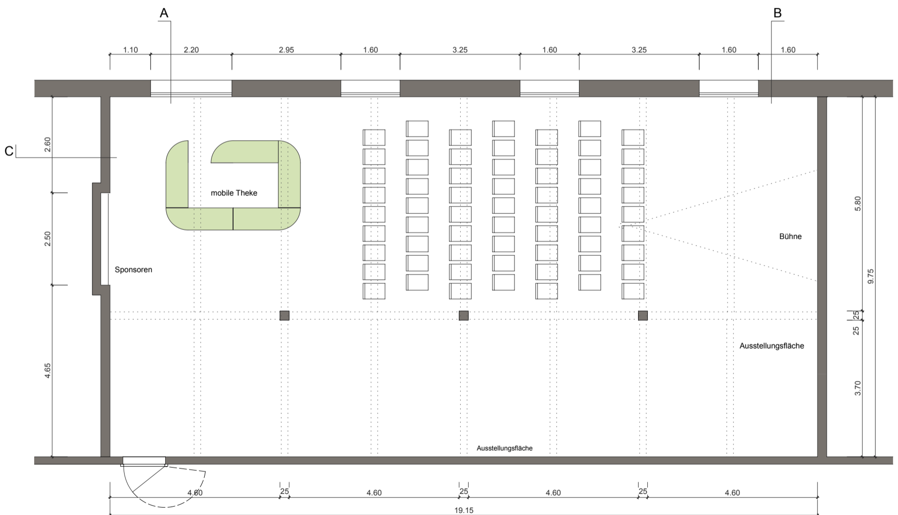
Grundriss Veranstaltungsraum
