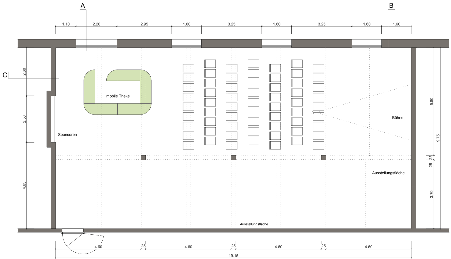
Grundriss Veranstaltungsraum
